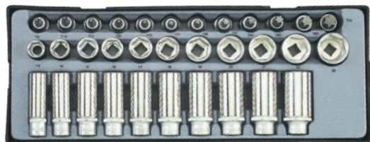
Module doppen 6 kant + torx 3/8" 33dlg Module de douilles 6 pans 3/8" + torx 33pcs 13-24mm T8-T60
