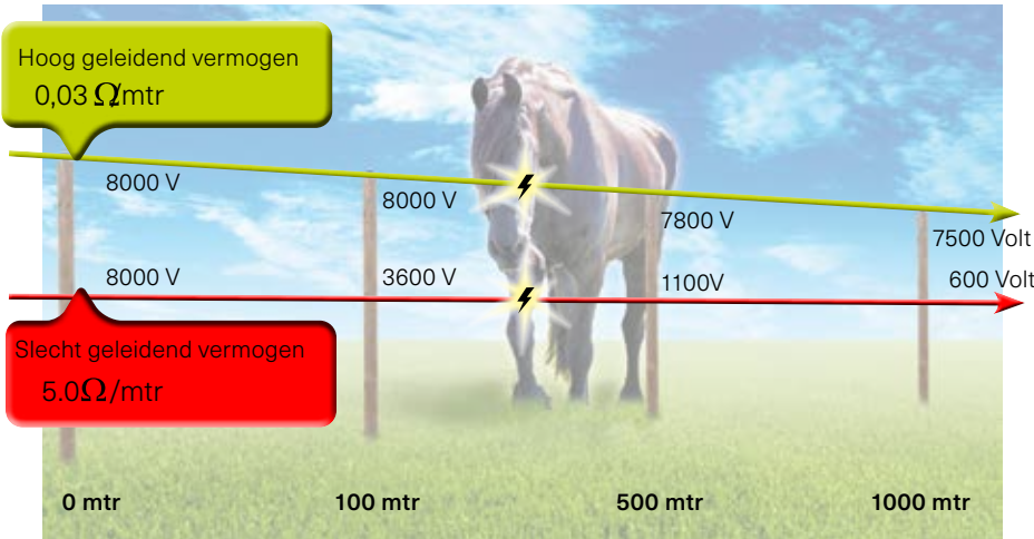
Voorbeeld aanduiding verschil in geleidend vermogen. Vanaf 1.500 Volt is een schok enigszins voelbaar voor dieren.
